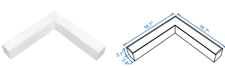
ILA-LDIDC(30)-8AK
