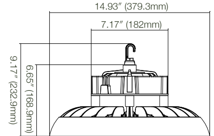
RHX-200 & 240
