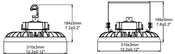
RWUX-(240/200/150)
