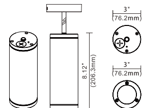
Pendant Mount
